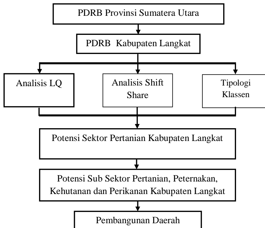
Gambar 2.2 Kerangka Pikir
