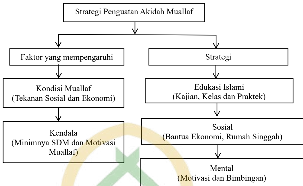
Gambar II.1 Kerangka Berpikir
