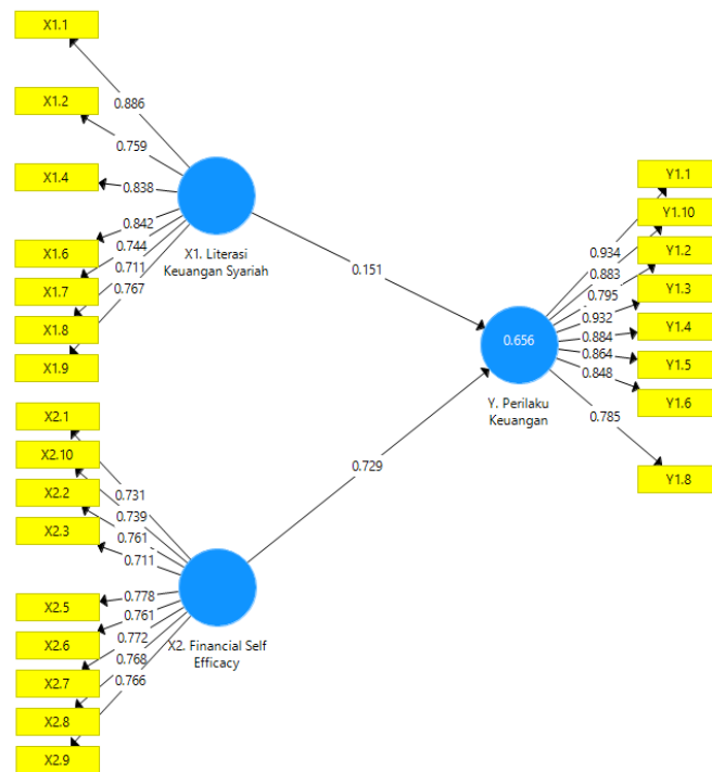
Gambar IV.5 Nilai Factor Loading (Modifikasi)
