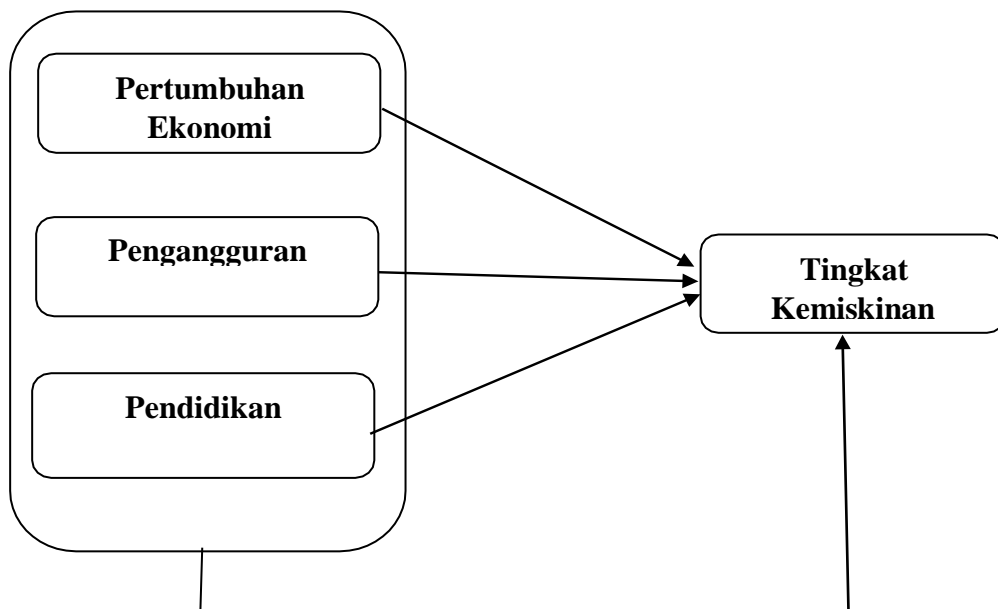
Gambar III.1 Kerangka pikir
